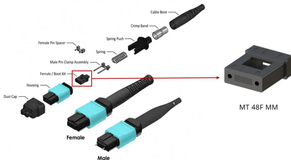
圖表三、光纖連接器及 MT Ferrule 示意圖
