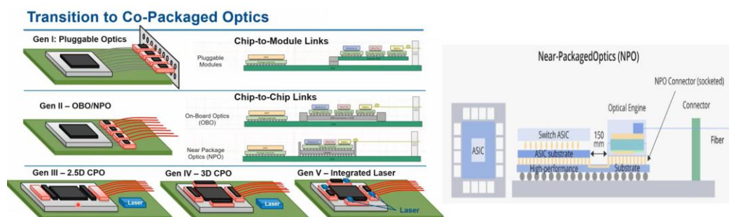
圖表四、CPO 技術路徑及 NPO 架構
